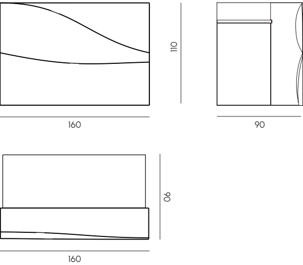
Baraonda modulo lineare Baraonda straight element
