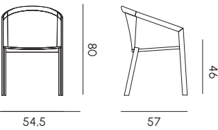
Poltrona da pranzo con schienale Dining armchair with fabric backrest
