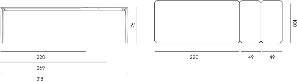
Tavolo da pranzo allungabile 100 x 220 Extendible dining table 100 x 220
