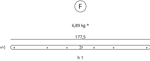
Barre di unione / Linking plates
