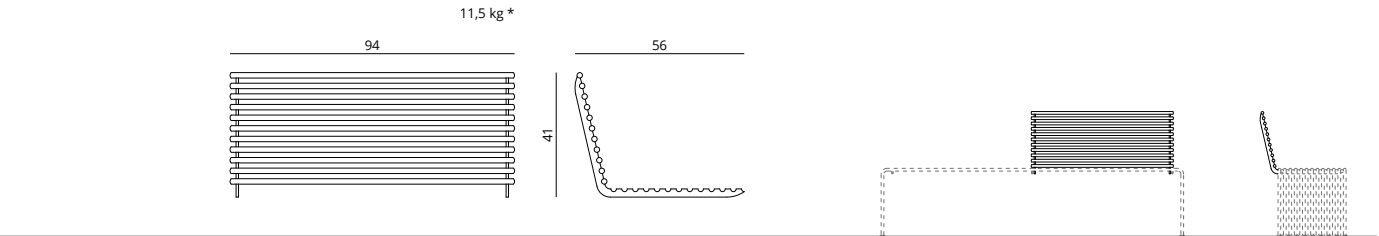
Schienale singolo panca piana / Single backrest flat bench
